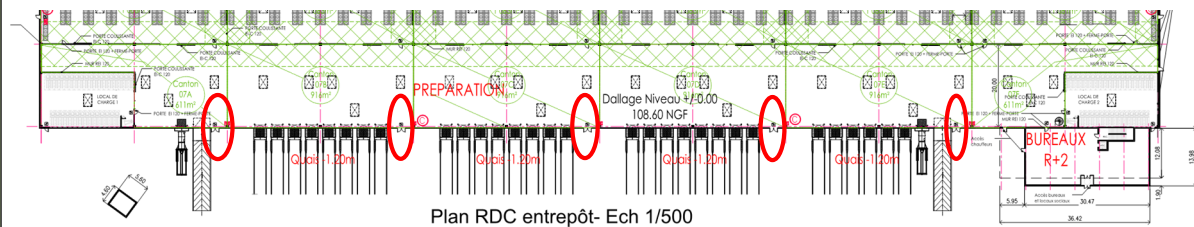
Plan RDC entrepôt- Ech 1/500
